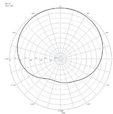
Polardiagramm @ 1 kHz
